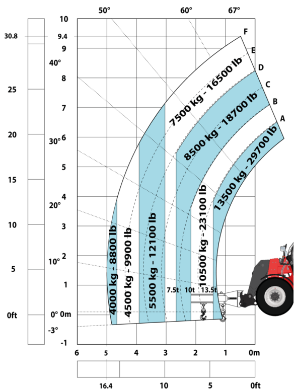
Машина на колесах с краном с 3-мя крюками 13500кг, метрическая система мер
